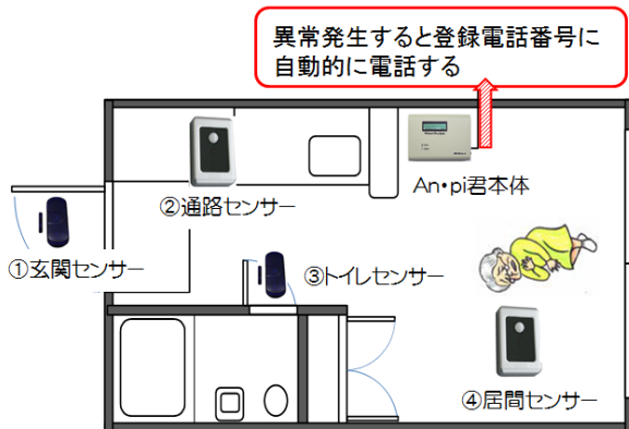
【平成 23 年度採択事業】 集合住宅用一人暮らしを見守る 安否確認システム「An・Piくん」 (株式会社エー・エス・ブレインズ)
